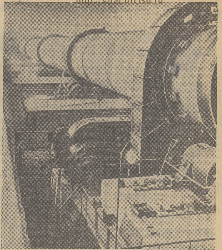
АРХАНГЕЛЬСКАЯ ОБЛАСТЬ. Вступила в строй действующих первая вращающаяся печь обжига клинкера на Савинском цементном заводе. Ее мощность — 310 тысяч тонн цемента в год. НА СНИМКЕ: первая печь обжига клинкера. (Фотохроника ТАСС).
