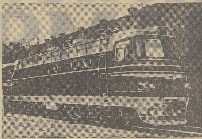
ЧЕХОСЛОВАКИЯ. Успешно проходит испытания новый локомотив 52-Е, заказанный Советским Союзом. Шесть двигателей мощностью 5 тысяч киловатт дадут возможность обеспечить скорость 160 километров в час.
