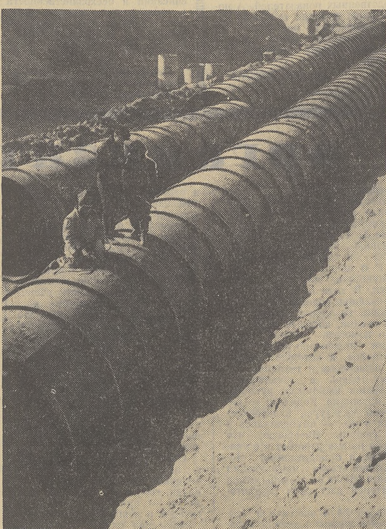
КАРАКАЛПАКСКАЯ АССР. В низовьях Ачу-Дарин развернулось строительство третьей очереди Ташкентской ГРЭС. К правднику Велико-Октябрь заработает первый ее блок. С вводом в строй всех агрегатов ГРЭС станет крупным энергетическим центром автономной республики. Ток от нее получат также промышленные предприятия северных районов Туркмени и Хорезмской области. НА СНИМКЕ: монтаж напорных циркуляционных водоводов. Фото А. Ходякова. (Фотохроника ТАСС).
