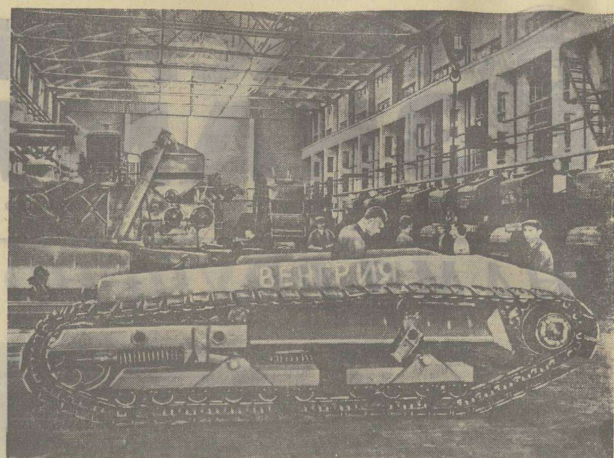
Самоходные гусеничные комбайны с маркой биробиджанского завода «Дальсельмаш» завоевали признание у хлеборобов Дальнего Востока. Заинтересовала машина и наших зарубежных друзей. НА СНИМКЕ: сборка комбайна, предназначенного для отправки в Венгрию. Фото Г. Хренова. (Фотохроника ТАСС).
