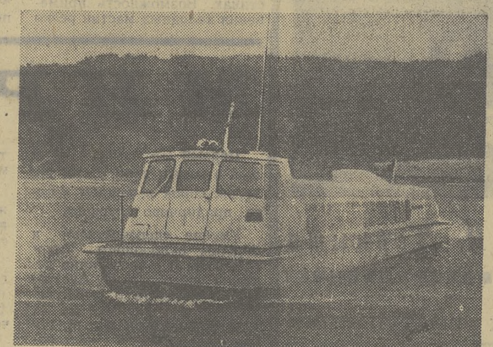
ГОРЬКИЙ. Новое судно на воздушной подушке «Горьковчанка», спроектированное ЦКБ «Волгоградспудопроект», предназначено для мелководных рек и способно развивать скорость 30-35 километров в час, имея на борту 48 пассажиров. «Горьковчанка» не нужно причалов и пристаней: для высадки пассажиров он сам «выходит» на берег. НА СНИМКЕ: «Горьковчанка» выходит на берег. Фото В. Войтенко. (Фотохроника ТАСС).
