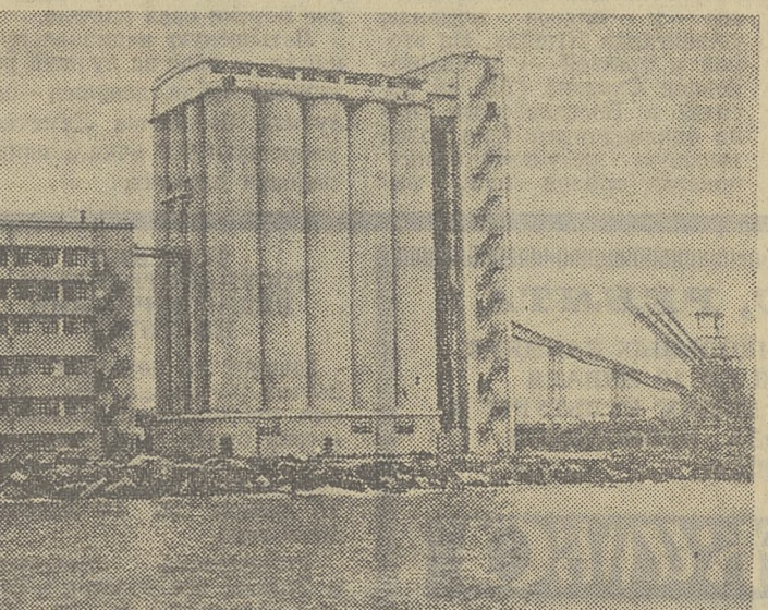
В столице Цейлона городе Коломбо с экономической и технической помощью Советского Союза построен крупный мельничный комбинат производительностью 235 тонн зерна в день. При комбинате имеется зернохранилище емкостью 20 000 тонн.
