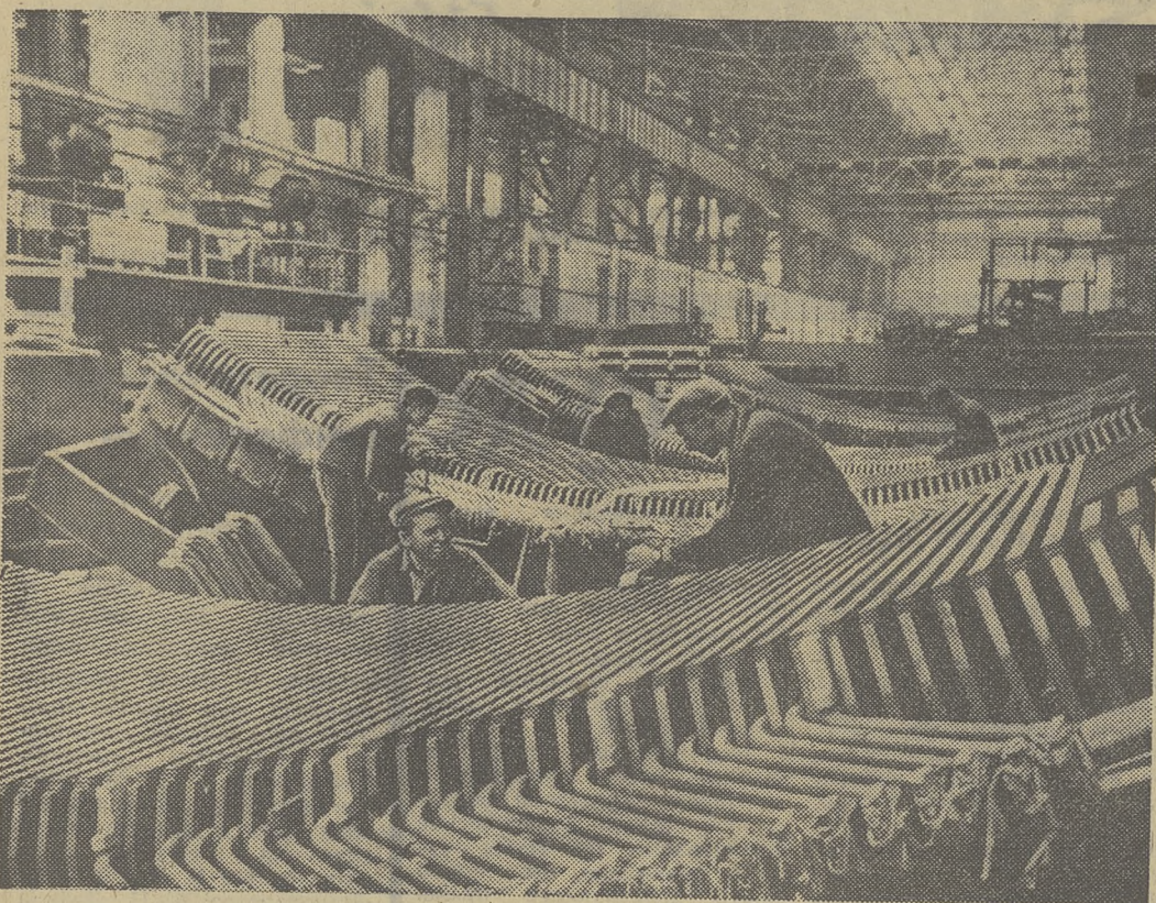
ЛЕНИНГРАД. Государственный «Знак качества» присвоен гидрогенераторам мощностью 175 тысяч киловатт. Они спроектированы в Ленинградском филиале Всесоюзного научно-исследовательского института электромеханики и изготовлены в объединении «Электросила».
