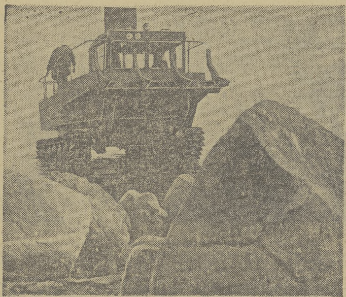
ПЕТРОЗАВОДСК. Государственной комиссией закончены испытания плавающего тракторного агрегата «ПТ-90», созданного конструкторами Онежского тракторного завода. Основное назначение машины — скатывание древесины в воду и на лед, установка рейдовых сооружений, разборка заломов и т. п. «Онежки» с успехом заменяют ледовые и водометные моторы. Годовой экономии от применения его на лесоплаве составляет от 9 до 14 тысяч рублей. Фото К. Бена.
