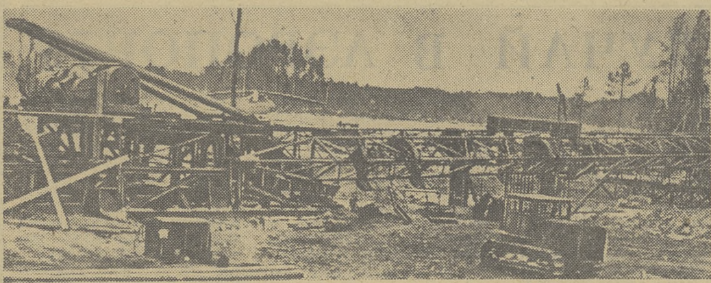
На снимках: БУ-125БД пока еще лежит на земле; вышкомонтажник (слева направо): Николай Тимофеев, Виктор Муравьев, Николай Алексеев. Вот они на снимке вместе со своим бригадиром Иваном Тереховым.
