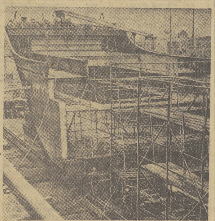
ПОЛЬША. Границные судостроители впервые провели в доке интересную операцию — удалили по просьбе заказчика судно и таким образом вдвое увеличили его грузоподъемность. Своеобразная «операция» длилась ровно месяц. Теплоход поместили в сухой док, разрешили поперек на две половины, раздвинули и «вышли» между ними новую секцию длиной 13 метров. НА СНИМКЕ: теплоход «Гейша», разрезанный на две части. (Фото АФ-ТАСС).
