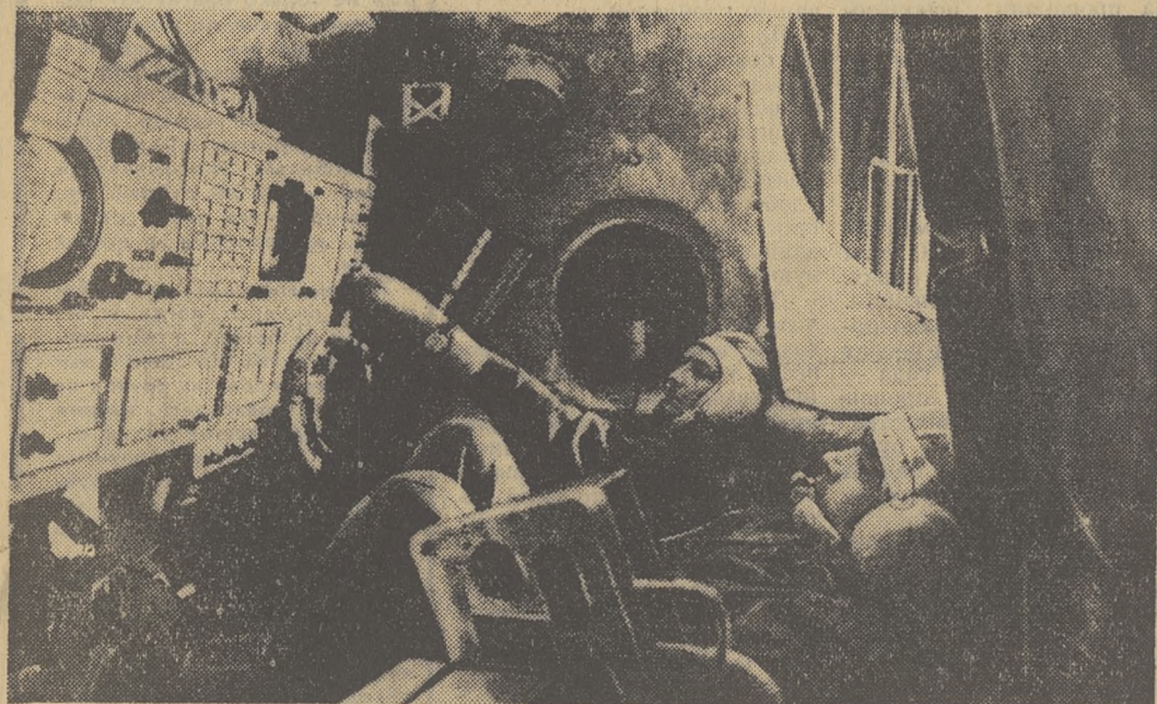
Командир космического корабля «Союз-9» А. Г. Николаев (на переднем плане) и бортинженер В. И. Севастьянов на тренировках. Фото В. Мусалына. (Фотохроника ТАСС).
