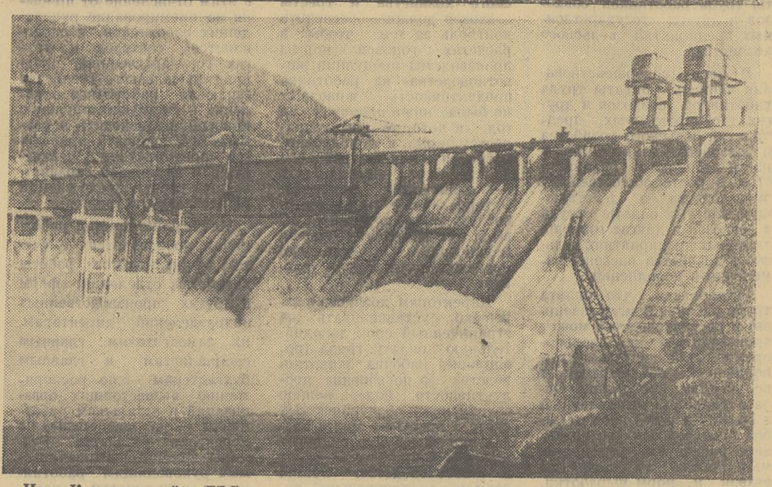
На Красноярской ГЭС проводятся испытания водосливной части исполненной плотины, что пере-
