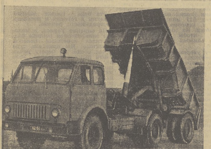
БОЛОРУССКАЯ ССР, МАЗ-504-Г и МАЗ-511-А — новые машины, созданные коллективом минских авто- мобилостроителей на базе МАЗ-500. Они предназначены для перевозки зерна, а также строительных материалов. Грузоподъемность машины МАЗ-504-Г с полуприце- пом — 14 тонн, а МАЗ-511-А с прицепом — 16 тонн. Обе автомашины снабжены двигателями в 180 лошади- ных сил, скорость их 75 километров в час. Разгрузка кузовов производится водителями из кабины. Фото В. Лупейко. Фотохроника ТАСС.
