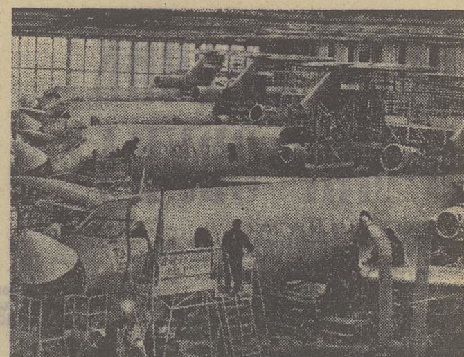
Самолетостроители Саратовского авиационного завода укладывают в самолет детали, узлы и агрегаты к реактивному лайнеру «ЯК-40» сдают с первого предъявления.
