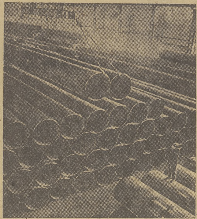
ЧЕЛЯБИНСК. Первые десятилетия эшелона стальных труб в 1971 году отправлены с Челябинского трубопрокатного завода. Они пойдут на сооружение газопроводов и нефтяных магистралей. За последние годы выпуск продукции на предприятии за счет повышения производительности труда вырос почти на треть. Впервые здесь освоено изготовление стальных газопроводных труб диаметром 1220 миллиметров. Только один цех электросварных изделий большого диаметра дал за пятнадцать месяцев 40 тысяч километров труб — на целую длину эшелона. НА СНИМКЕ: участок отгрузки труб большого диаметра. Фото В. Клиниченко. (Фотокорреспондент ТАСС).
