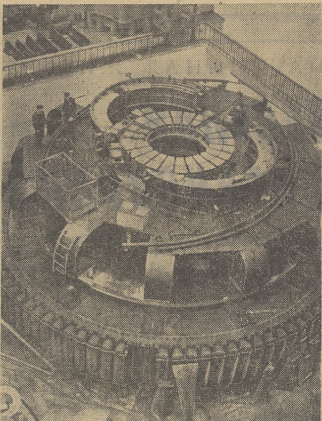
НОВОСИБИРСК. В машинном зале Новосибирской ГЭС установлено 7 гидроагрегатов общей мощностью 400 тысяч киловатт.
