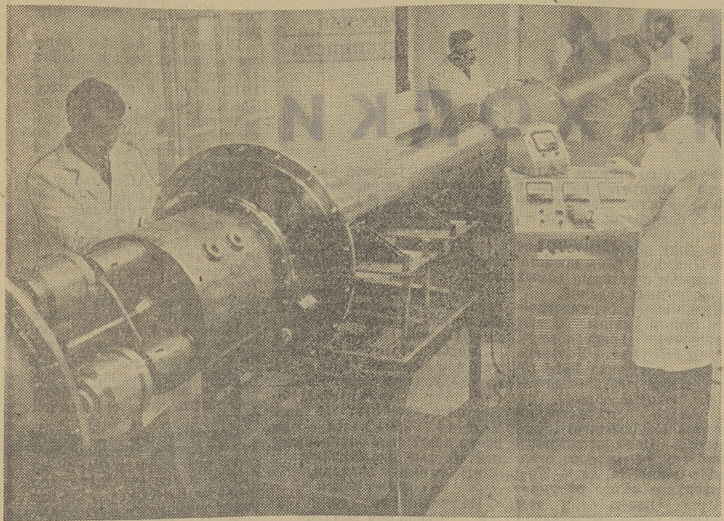
МОСКВА. В ближайшее десятилетие для транспортировки больших потоков электроэнергии потребуются принципиально новые виды линий электропередач. Ученые и конструкторы Энергетического института имени Г. М. Кржижановского разрабатывают и испытывают первую в Советском Союзе модель трехфазного сверхпроводящего кабеля. Внедрение в народное хозяйство сверхпроводящего кабеля откроет широкие возможности передавать энергию от электрических
