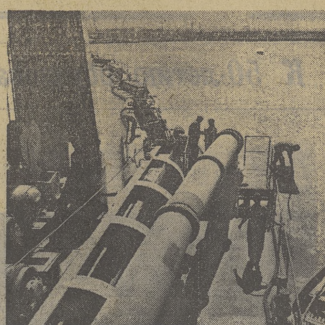
УЗБЕКСКАЯ ССР. На строительстве Тахташатской ГРЭС. Прокладка нового русла Амударьи. Здесь работает первоклассная отечественная гидротехника.
