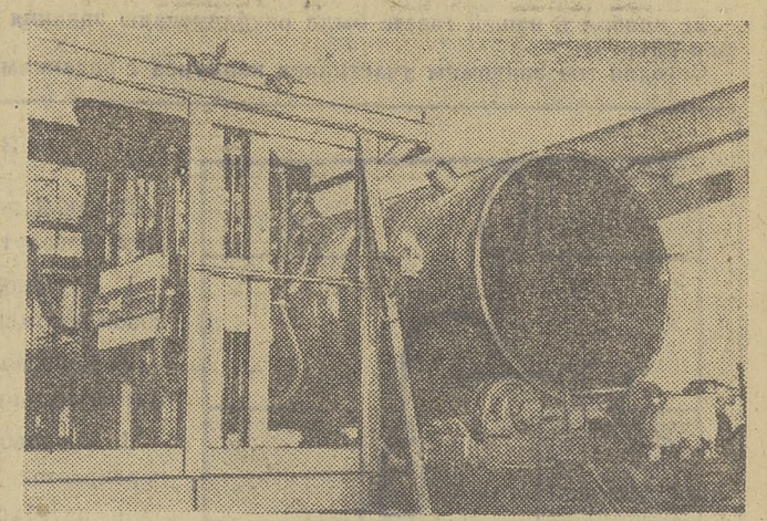
НА СНИМКЕ: бета-лучевой дефектоскоп для контроля сварных швов. Вы не видите здесь операторов, и это не случайно, потому что весь контроль за качеством толстолистовых сварных конструкций производится автоматически. Конструкция новой установки, которая уже используется на Ижорском заводе имени Ижоры, разработана под руководством профессора В. И. Горбунова.
