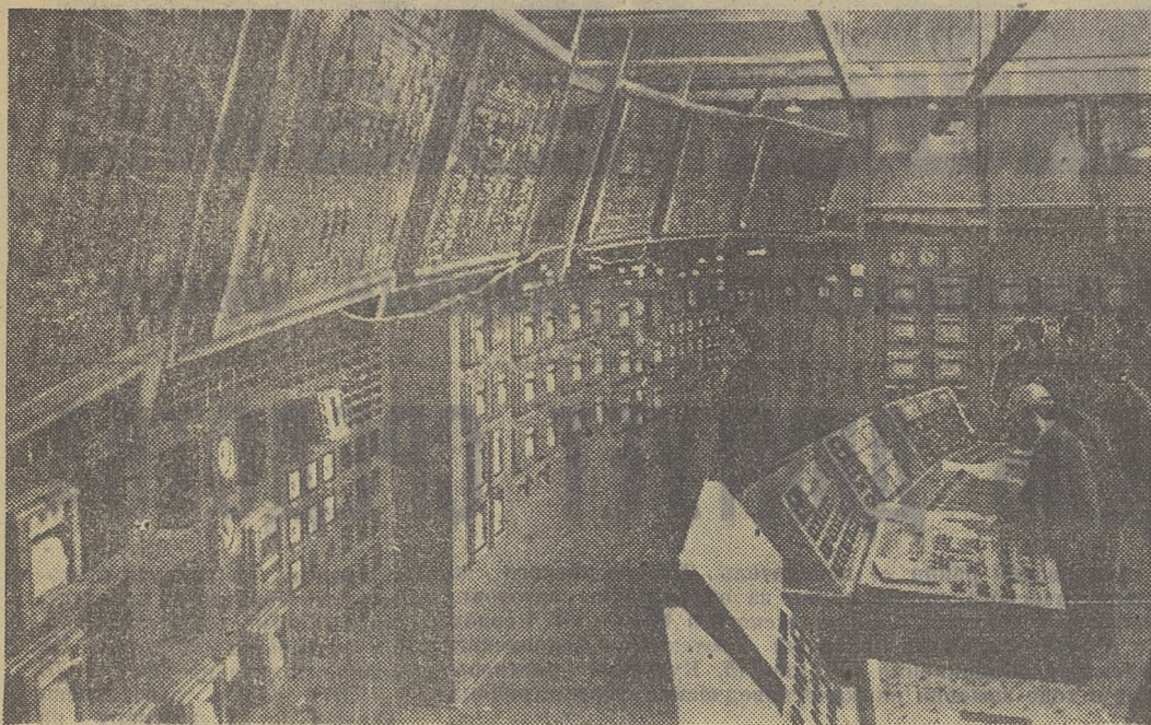
Первый агрегат Рязанской ГРЭС дал промышленный ток.
