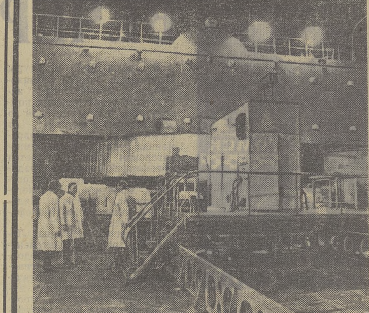
Широкий комплекс работ по изучению микромира осуществляется в Ленинградском институте ядерной физики имени Б. П. Константинова, одном из самых молодых академических научных центров. Проводя фундаментальные исследования по физике элементарных частиц и структуре ядра, ученые осуществляют уникальные эксперименты на синхротроне — ускорителе элементарных частиц, мощном реакторе и оригинальных установках, созданных в институте. Интересные работы ведутся здесь и по изучению процессов научных исследований с широким применением электронно-вычислительной техники.
