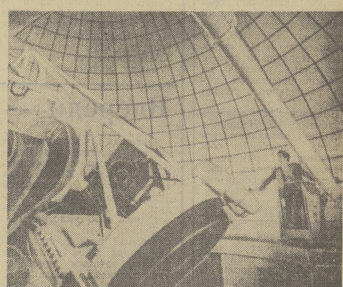
АРМЯНСКАЯ ССР. Один из главных астрономических приборов Бюраканской астрофизической обсерватории — телескоп с диаметром зеркала 2,6 метра (ЗТА-2,6).
