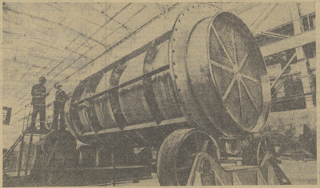
РОСТОВСКАЯ ОБЛАСТЬ. Эффективно трудится коллектив таганрогского завода «Красный котельщик», где производится оборудование для тепловых и атомных электростанций страны и на экспорт. Здесь нет отставания цехов, участков, бригад. НА СНИМКЕ: на сборочном стенде нового цеха теплообменной аппаратуры за-
