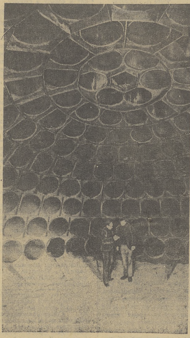
УКРАИНСКАЯ ССР. Под Киевом строители треста Промтехмонтаж-2 смонтировали уникальную трубчатую взрывную камеру. Она предназначена для проведения научных экспериментов в области получения и обработки новых материалов с использованием зарядов взрывчатого вещества весом до 200 килограммов.
