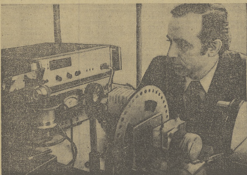
Старший научный сотрудник В. Б. Ахманаев изучает свойства полупроводникового материала с помощью созданного в СФТИ прибора ИПК-1, удостоенного серебряной и бронзовой медалей ВДНХ в 1977 году. Фото М. Уразова.
