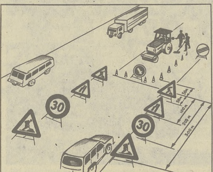
Ограждение участка работ на внутренней полосе движения.
