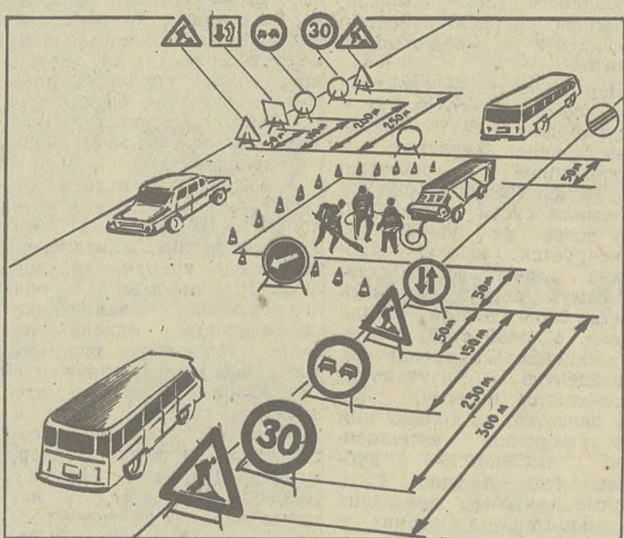
Ограждение участка работ на дороге с двумя полосами движения.
