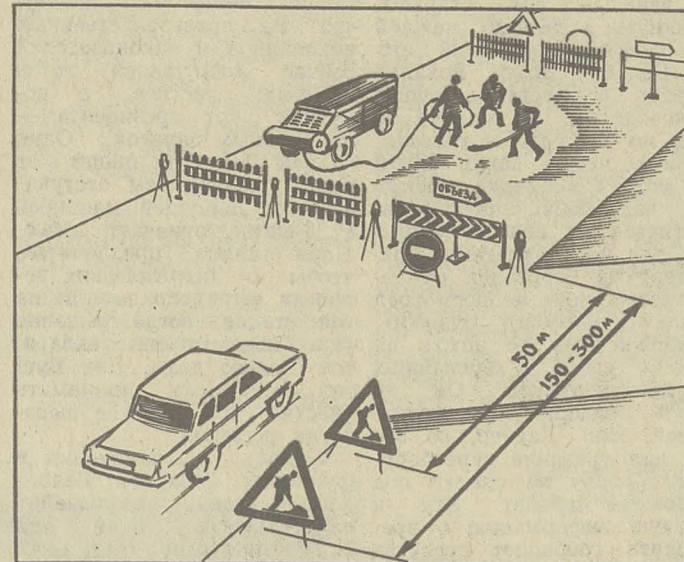
Ограждение участка дороги по всей ширине проезжей части.
