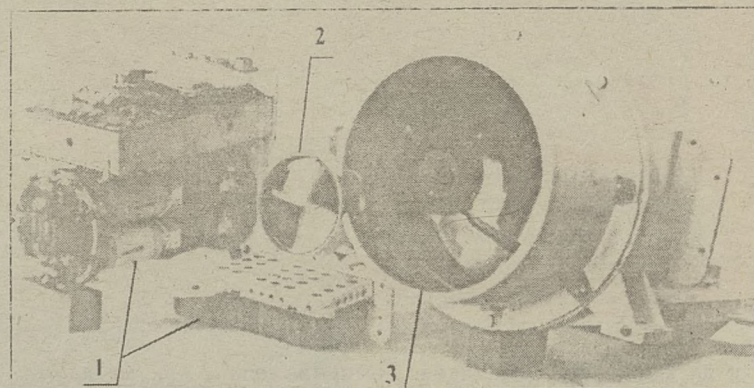
НА СНИМКЕ: космический лидар «Балкан-1»: 1 - лазер с блоком питания, 2 - оптическая антенна передатчика, 3 - приемный объектив лидара.
