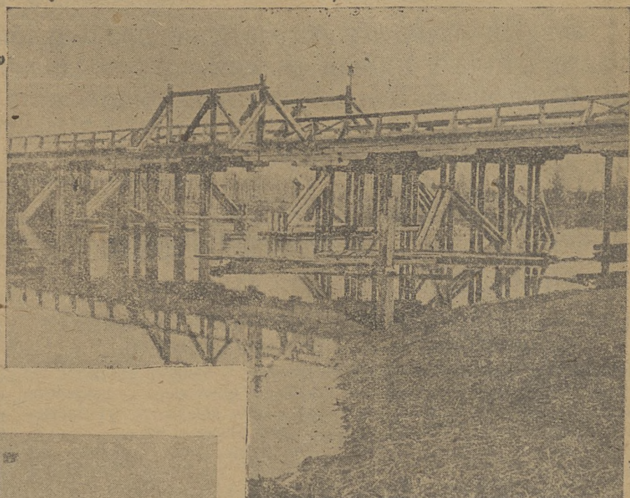
Мост через р. Тару в поселке Кордонском (Биаза), построен в мае 1928 года. Стоит около 8 тысяч рублей
