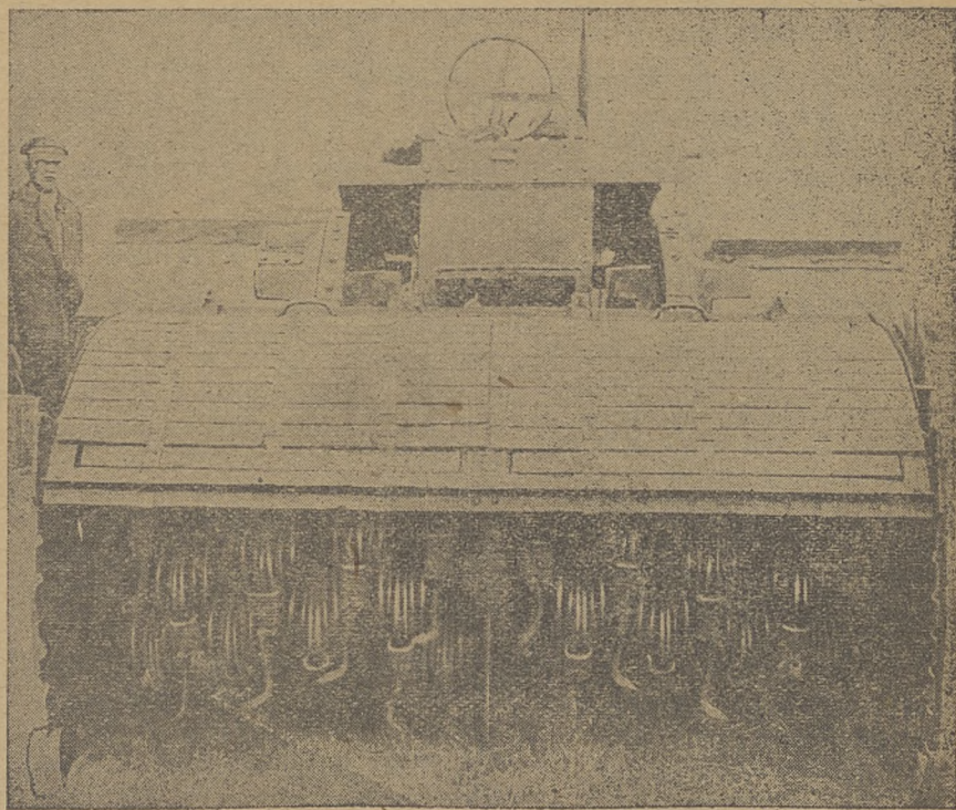
Вид почвенного фрезера сзади. На переднем плане фрезерная коробка с режущими крючьями
